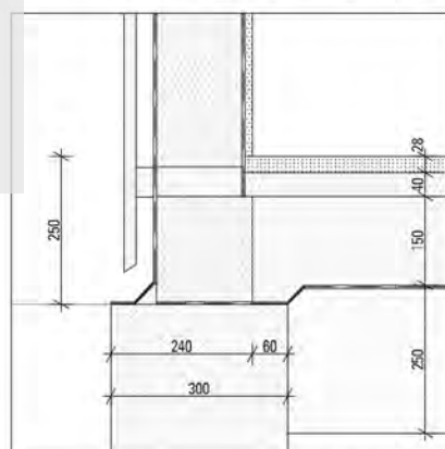
Fußpunkt Verkleidung
