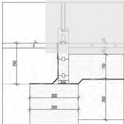
Fußpunkt Schiebetür
