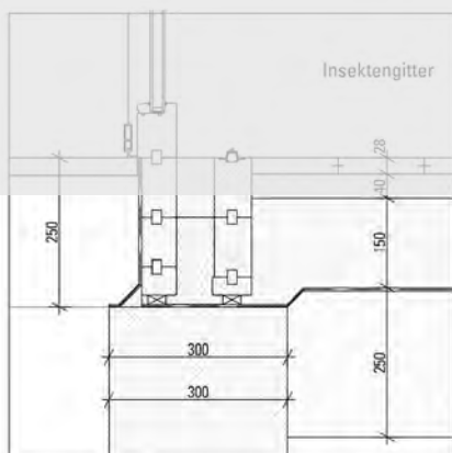
Fußpunkt Festverglasung
