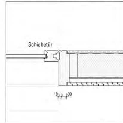
Horizontalschnitt Schiebetür
