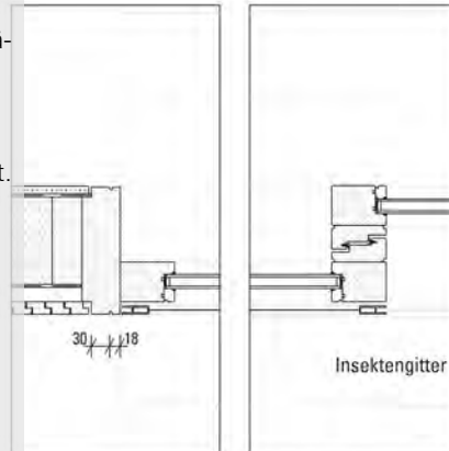
Horizontalschnitt Festverglasung
