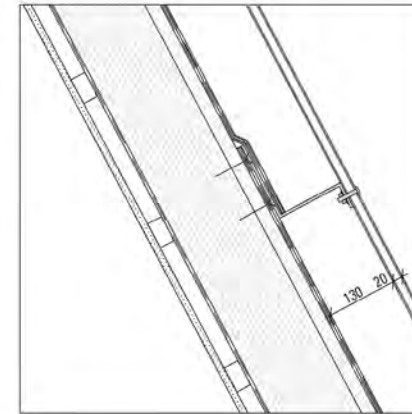
Rankgerüst Längsschnitt
